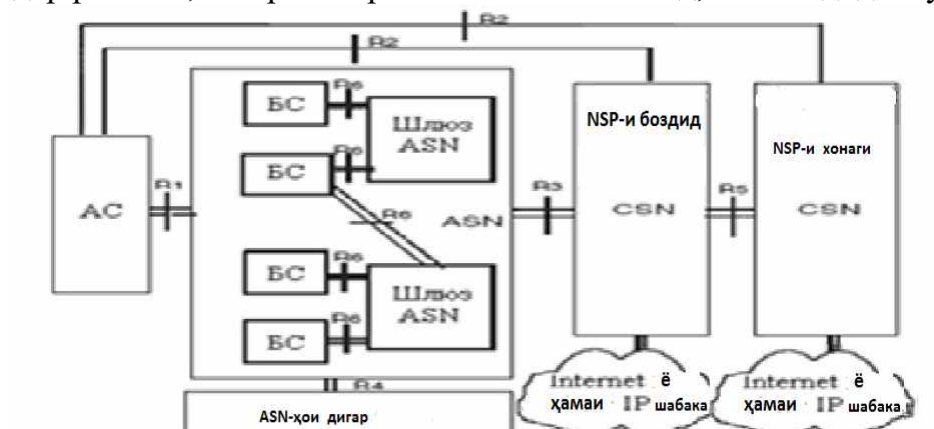
Расми 2. Модели асосии шабака.
