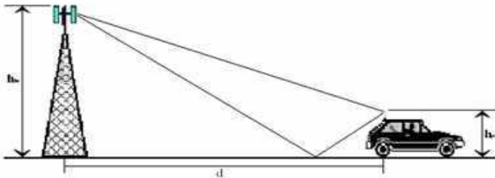
Расми 4. Паҳнкуни сигнали радиои дунура (двухлучевое).
